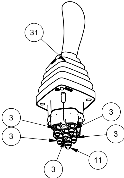
RH JOYSTICK
