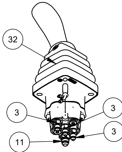
LH JOYSTICK
