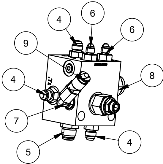
RH JOYSTICK
